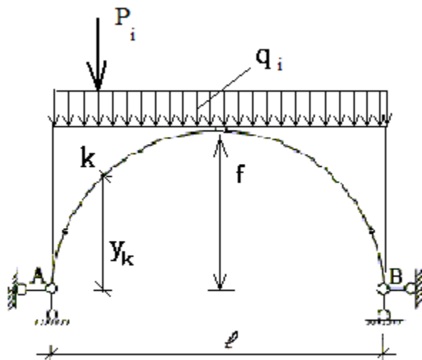
5-расм. Шарнирли арка
